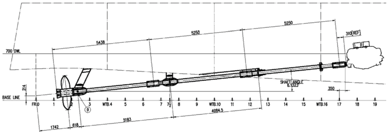
Figure 9 The direct propulsion shafting system [4] Slika 9 Sustav direktnog propulzijskog osovinskog voda [4]
