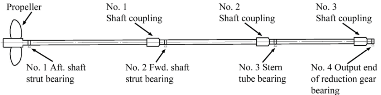
Figure 10 The illustration for direct propulsion shafting model Slika 10 Prikaz modela direktnog propulzijskog osovinskog voda
