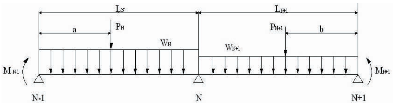
Figure 5 The illustration for shafting analysis using TMEM Slika 5 Prikaz analize osovinskog voda upotrebom metode TMEM
