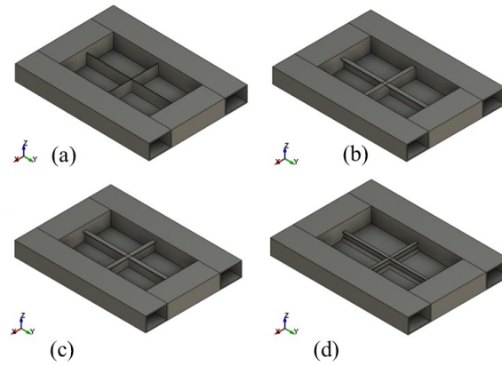
Fig. 11 Cross stiffener type geometry: (a) Cross-I, (b) Cross-L, (c) Cross-T, (d) Cross-Y
