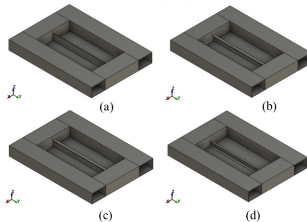
Fig. 10 Single stiffener type geometry: (a) Single-I, (b) Single-L, (c) Single-T, (d) Single-Y
