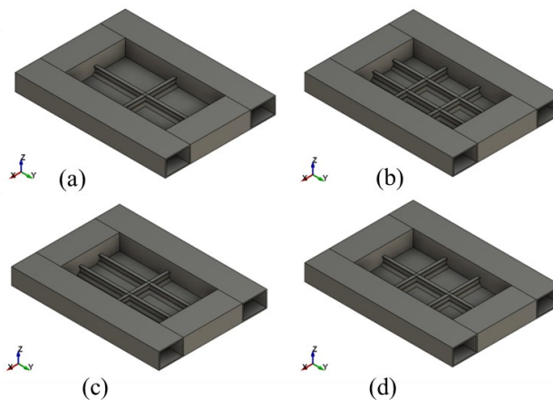
Fig. 13 Geometry of stiffener configuration: (a) Config. 1, (b) Config. 2, (c) Config. 3, (d) Config. 4
