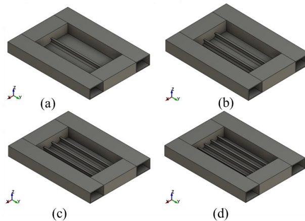
Fig. 12 Geometry of stiffener spacings: (a) Spacing 1, (b) Spacing 2, (c) Spacing 3, (d) Spacing 4
